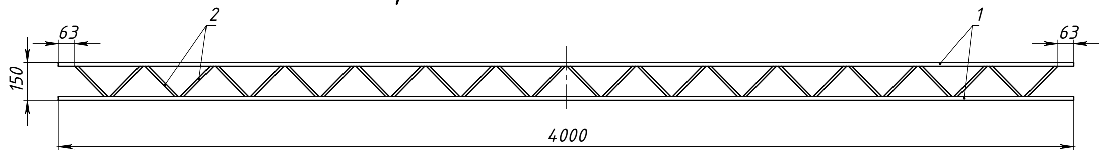
Ферма металлическая ФМ 150 L4м
